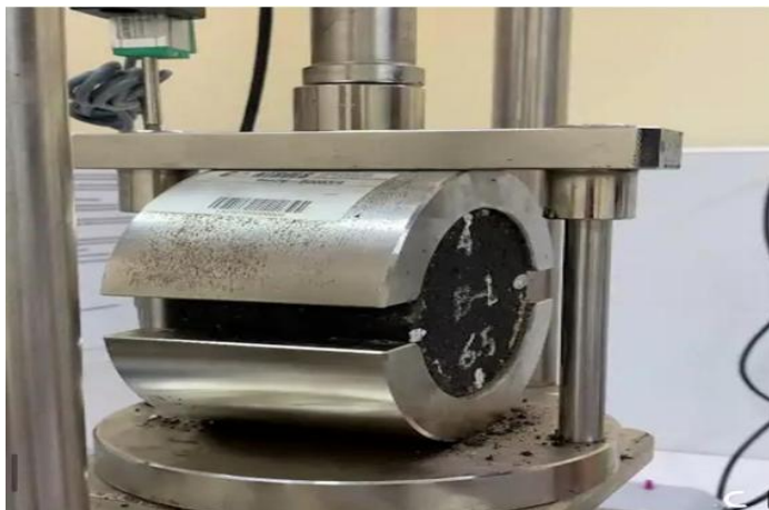
يوضح الشكل (5) اختبار مارشال.
